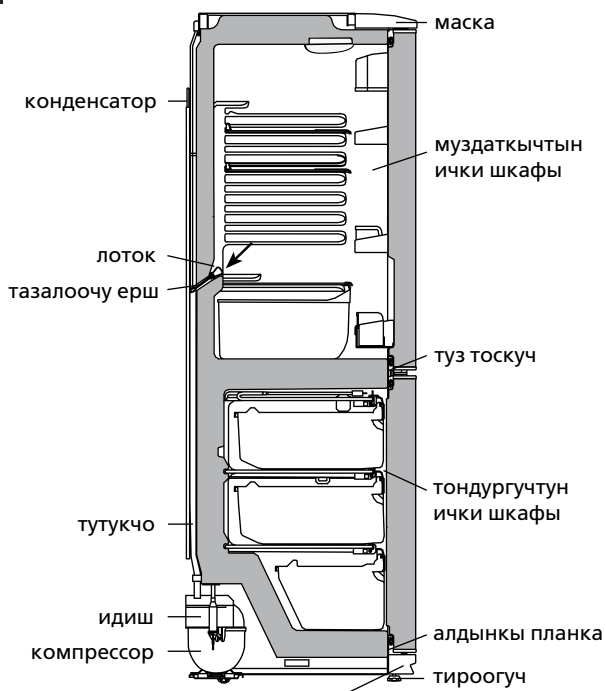
Сурот 4 – Муздаткычтан аккан суунун схемасы
