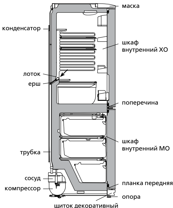
Рисунок 4 – Схема слива талой воды из XO
