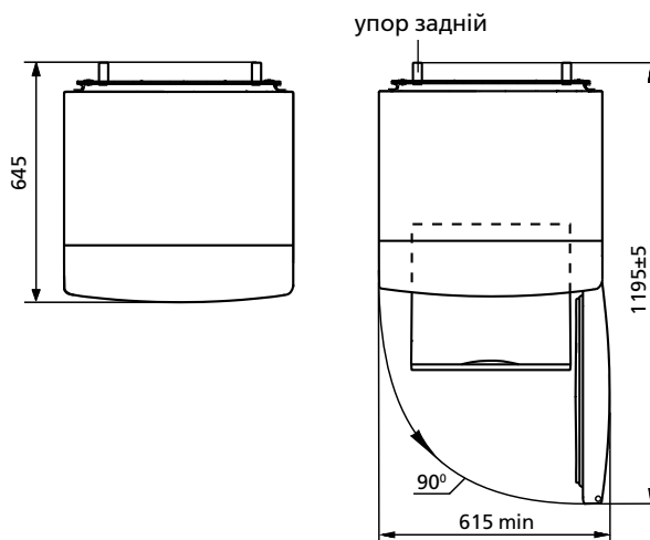
Рисунок 2 – Холодильник (вигляд зверху)
