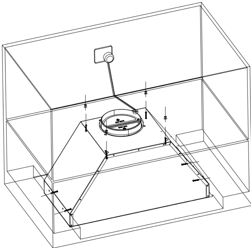
Рис 6. Вид сборки
