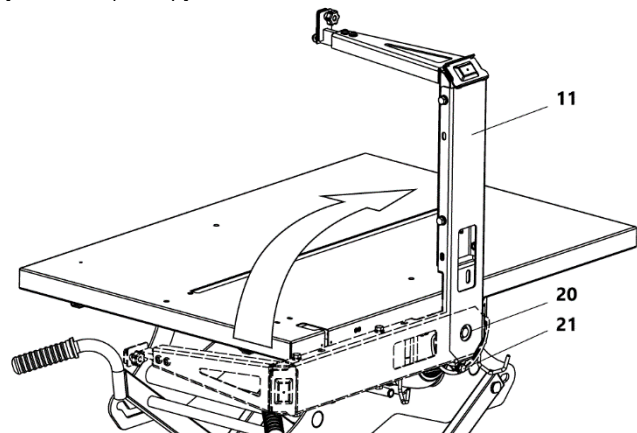
Рисунок 4 Установка стойки 11 – стойка; 20, 21 – болт
