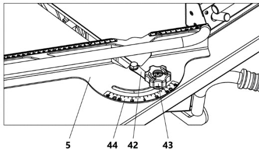
Рисунок 9 Установка упора под углом 5 – упор; 42 – указатель; 43 – ручка; 44 – шкала
