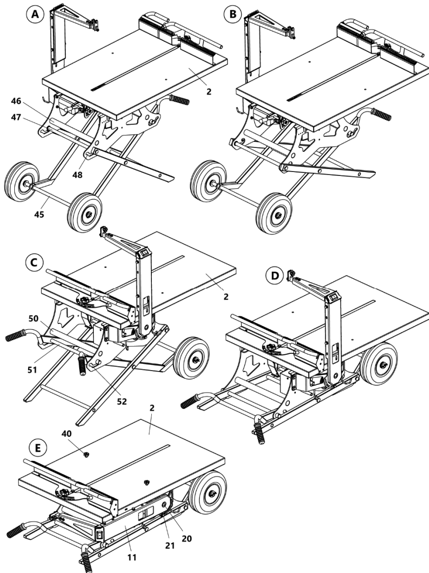
Рисунок 14 Общий вид станка в транспортном положении 2 – рабочий стол; 11 – стойка; 20, 21 – болты; 40 – винт транспортный; 45, 49 – поперечина; 46, 50 – труба; 47, 51 – ось; 48, 52 – зацеп
