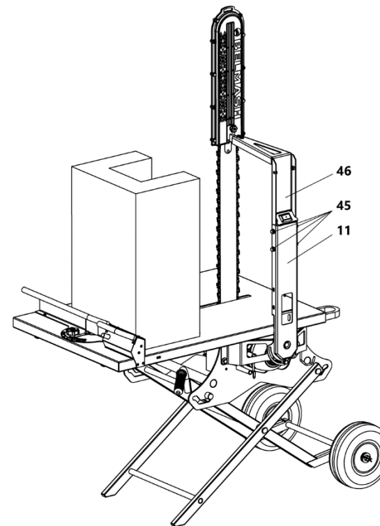
Рисунок 10 Общий вид станка с вырезанным U-блоком 11 – стойка; 45 – болт; 46 – кронштейн
