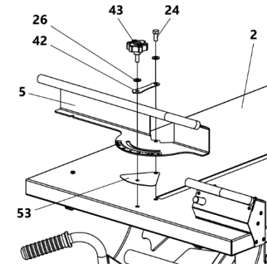
Рисунок 6 Установка упора 2 – стол; 5 – упор; 24 – болт; 26 – шайба; 42 – указатель; 43 – ручка; 53 – планка
