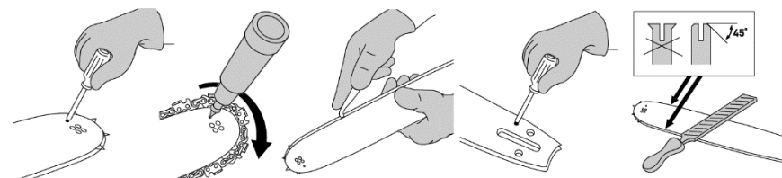
Рисунок 12 Обслуживание шины направляющей
