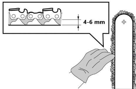
Рисунок 11 Проверка натяжения цепи
