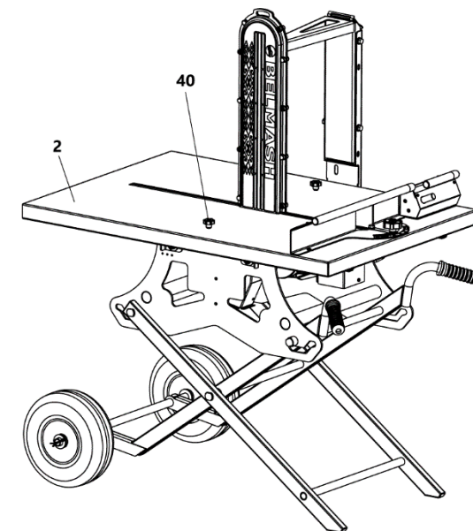
Рисунок 13 Общий вид станка в транспортном положении
