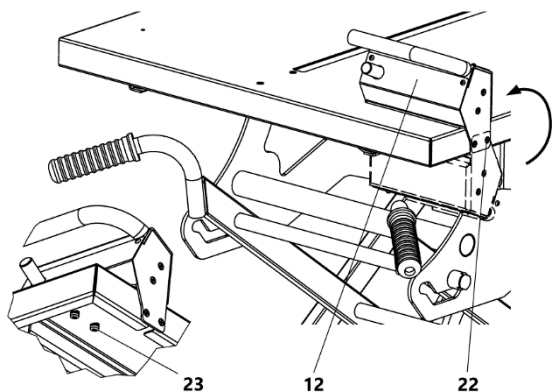
Рисунок 5 Установка пульта управления 12 – пульт управления; 22, 23 – винт
