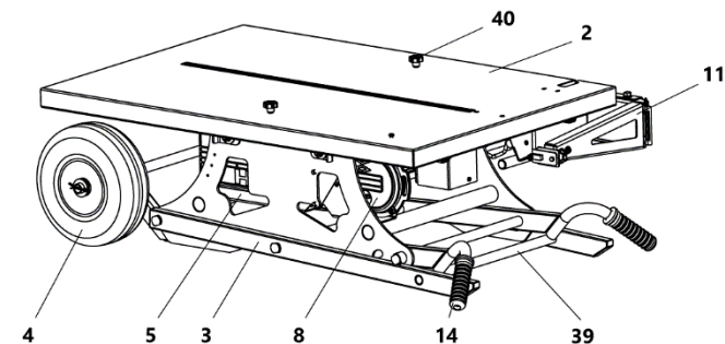
Рисунок 3 Общий вид станка в упаковке 2 – стол; 3 – опора; 4 – колесо; 5 – упор; 8 – кожух защитный; 11 – стойка; 14 – ручка; 25 – винт упорный; 39 – поперечина; 40 – винт транспортный
