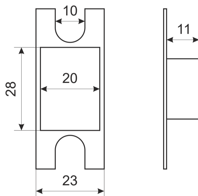
Пластиковая вставка
