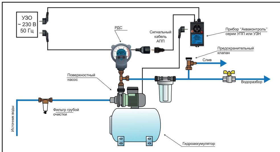
14.3 Пример подключения РДС к УЗН или УПП “Extra Акваконтроль” с применением АПП
