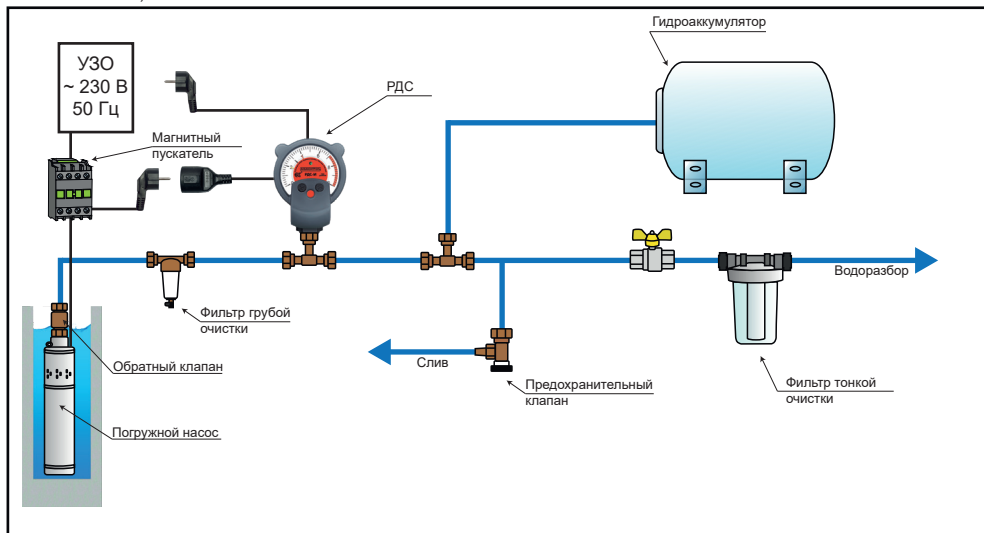
14.4 Пример подключения РДС к скважинному однофазному или трехфазному насосу мощностью более 1,5 кВт
