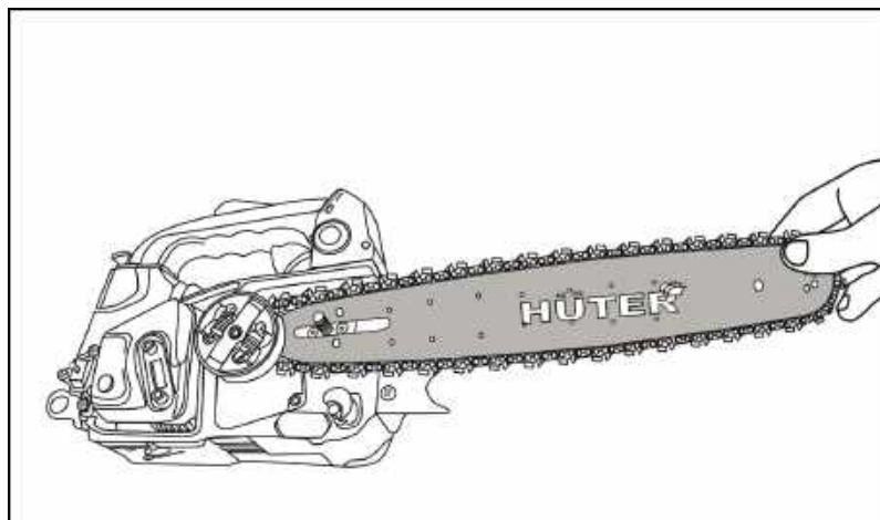
Рис. 6. Установка цепи
