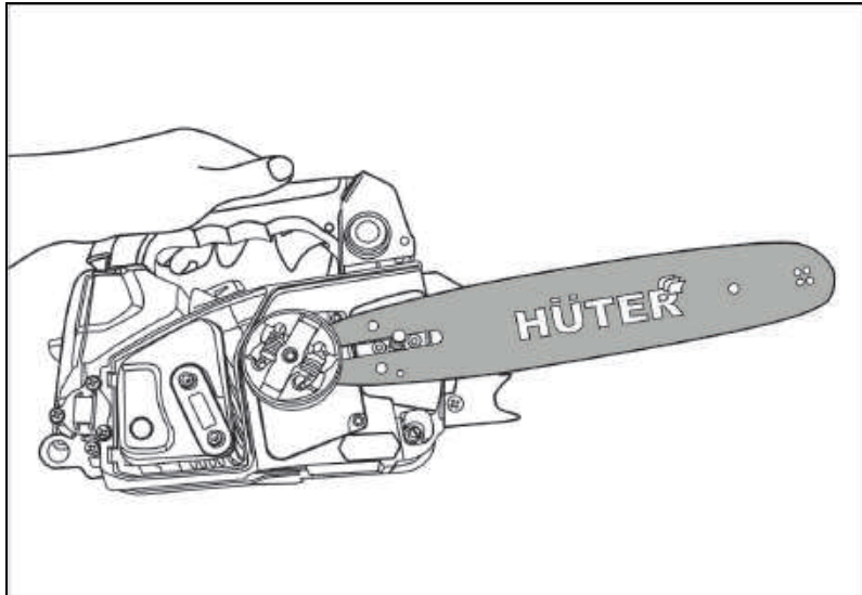
Рис. 5. Установка шины
