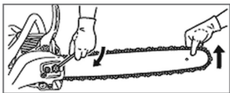
Рис. 4 Затяжка гаек крепления шины
