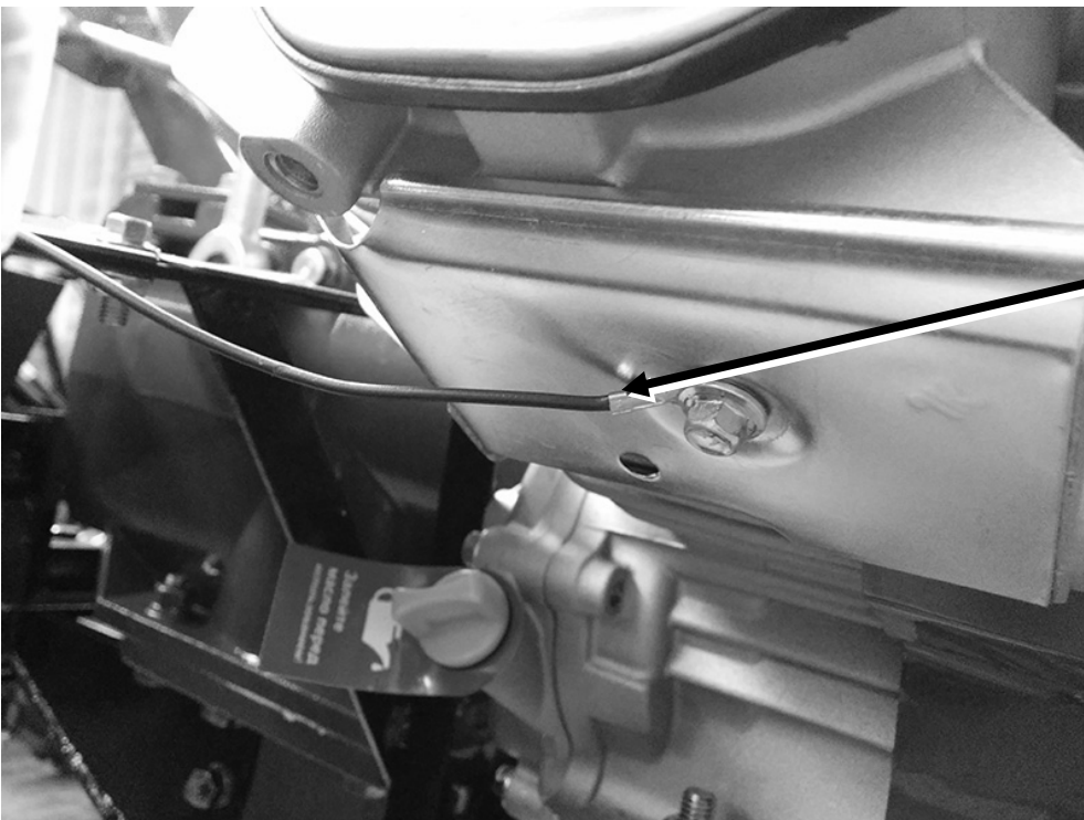
Кабель «масса»
