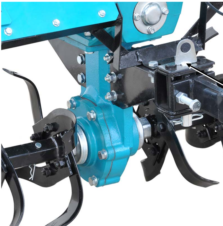
Стопорный палец
