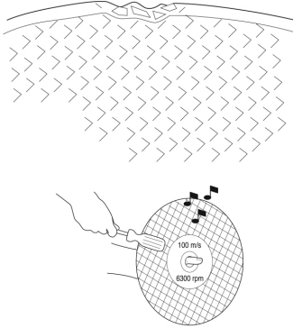
Рис. 10 Проверка абразивного диска
