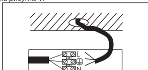
Рисунок 1. Клеммный зажим светильника
