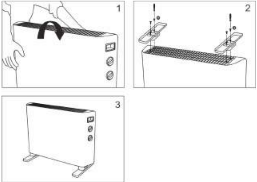
Рис. 1. Напольная установка
