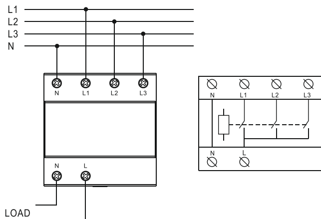
Рис.5. Схема подключения
