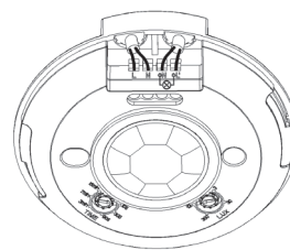
Закрытая установка
