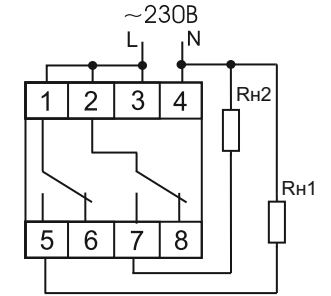
Рис.1 Рекомендуемая схема подключения таймера PCZ-527 и нагрузки к сети 230 В.
