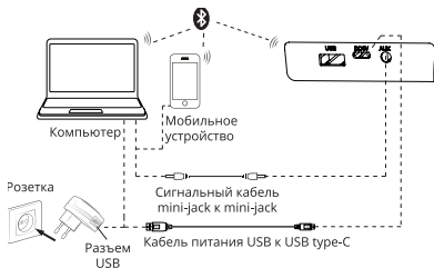
Рис. 2. Схема подключения
