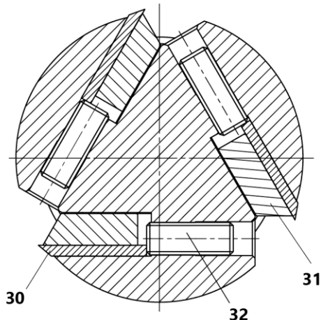
Рис. 11 Регулировочное устройство
