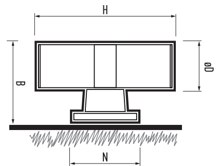
Рис. 2 Двухстороннее свечение
