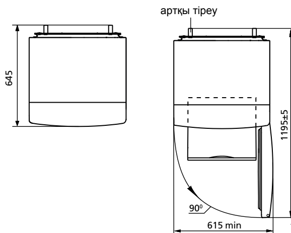
2 сурет – Тоңазытқыш (үстінен қарағанда)
