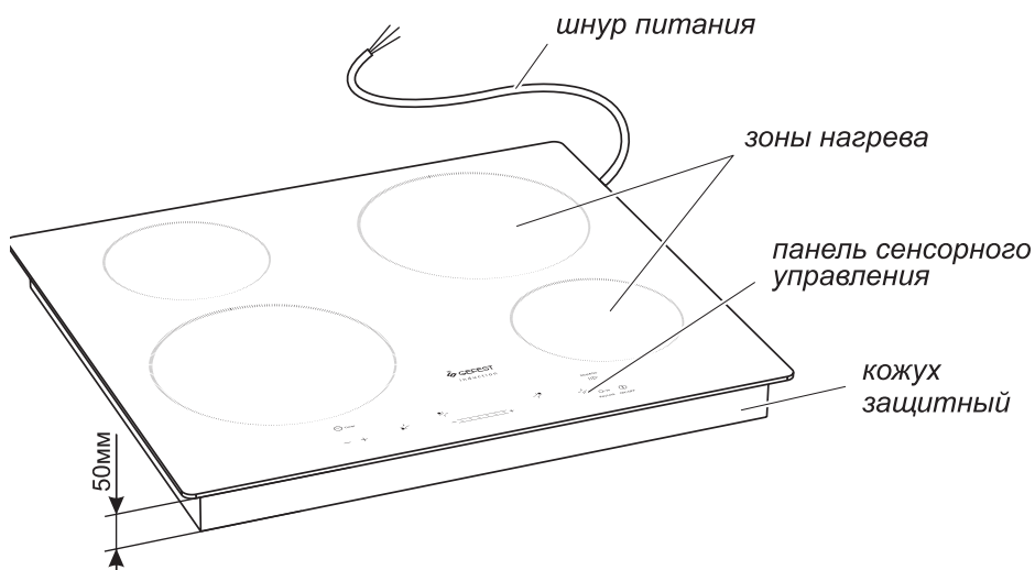
Рис. 1 Стол СН4232, СН4232 К32 (СН4232 К1; СН4232 К12)
