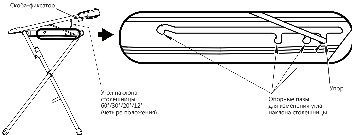
(рис. 5) Схема изменения наклона столешницы (арт. КНД4, КНД4П)
