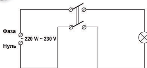
Схема подключения
