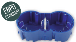
KE-501 Коробка двухместная для крепления выключателей и розеток 136x66x47,4 мм
