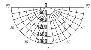
PWP-C6 PRO
