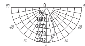
PTR 0728 28w 60°
