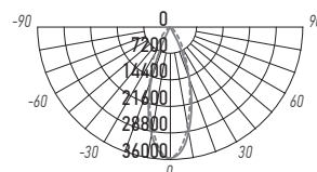
PTR 0620 20w
