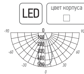
PSP-S 7w
