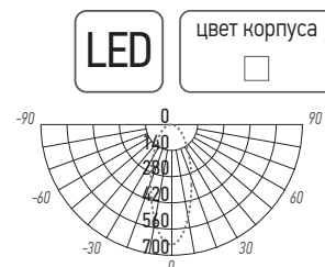
PSP-S 412 2x8w
