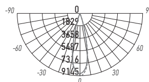
PTR 0728 28w 15°
