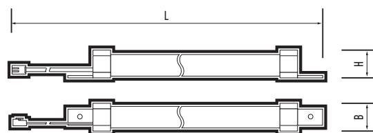
PEPP40-1.0H IP20. (Габаритные размеры аккумулятора)
