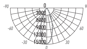
PTR 0325 25w
