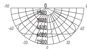
PPI-01 100w
