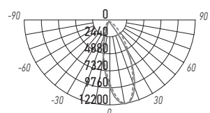
PTR 1615 15w
