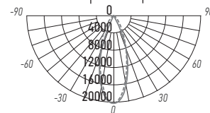
PTR 1335 35w
