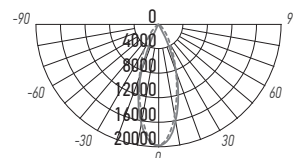
PTR 0530 30w
