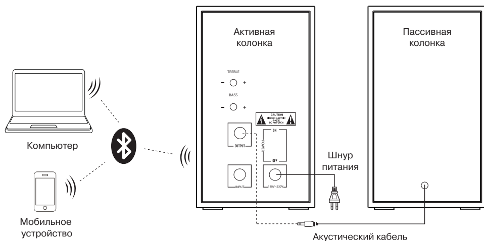
Рис. 3. Схема подключения источников аудиосигнала через Bluetooth-моуль
