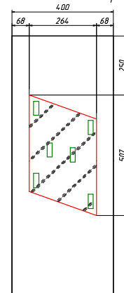
Схема наклейки зеркала
