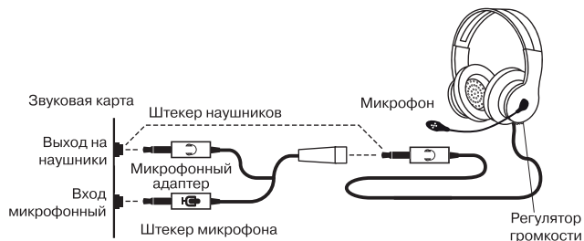
Рис. 1. Схема подключения
