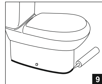
9 При необходимости нанести герметик в зазор между полом и унитазом.
