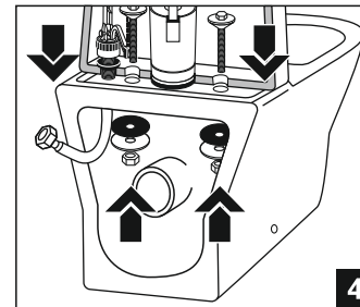
4 Зафиксировать бачок с помощью крепления к унитазу;
