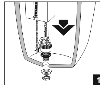
1 Установить в бачке наполнительную арматуру, согласно схеме монтажа поставляемой в комплекте арматуры;
