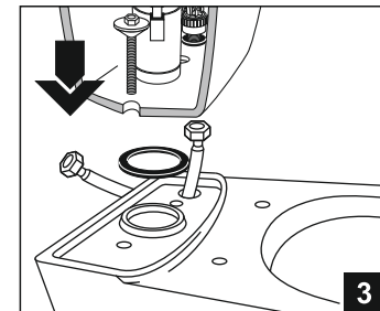
3 Надеть прокладку, установить бачок на полу унитаза, присоединить шланг водоснабжения к спускной арматуре;
