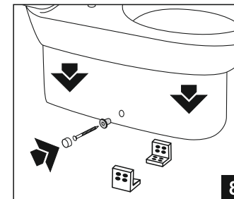
8 Закрепить унитаз согласно схеме, поставляемой в комплекте с креплением;
