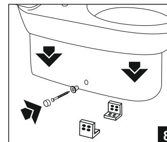
Закрепить унитаз согласно схеме, поставляемой в комплекте с креплением;
