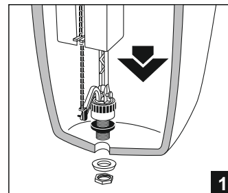
Установить в бачке наполнительную арматуру, согласно схеме монтажа поставляемой в комплекте арматуры;
