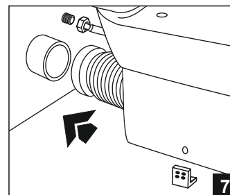
Разметить и закрепить КУС к полу. Подключить унитаз к канализации и системе холодного водоснабжения;
