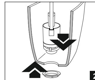
Закрепить в бачке спускную арматуру, согласно схеме монтажа поставляемой в комплекте арматуры;
