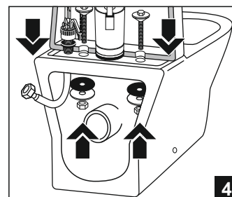
Зафиксировать бачок с помощью крепления к унитазу;
