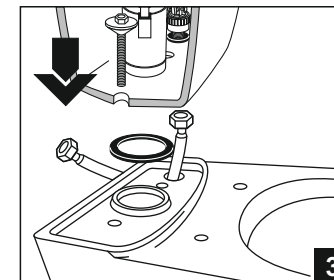
Надеть прокладку, установить бачок на полочку унитаза, присоединить шланг водоснабжения к спускной арматуре;
