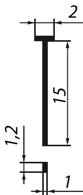
T-образный гвоздь
